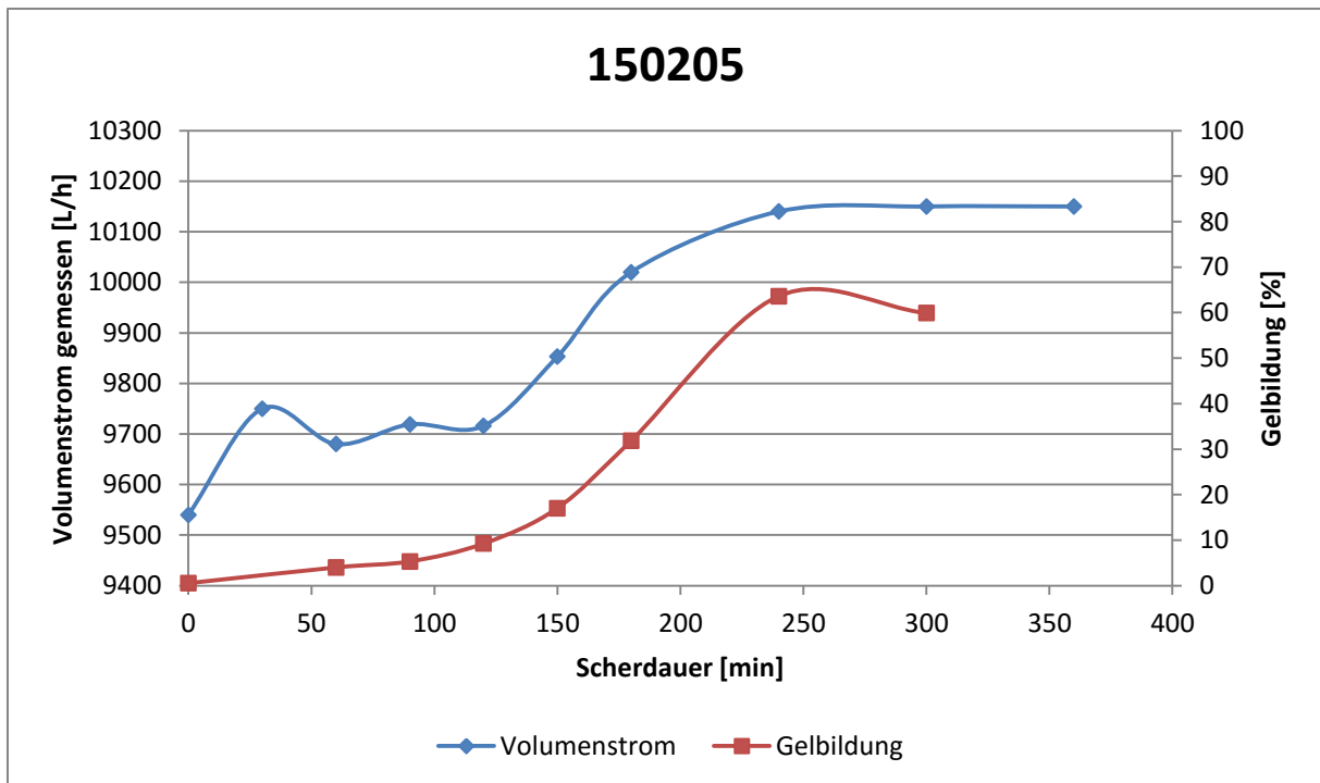
Abbildung 39: Volumenstrom und Gelbildung – normalsaugende Kreiselpumpe A, nominaler Betriebspunkt, \beta -Glucan-Charge #A02
