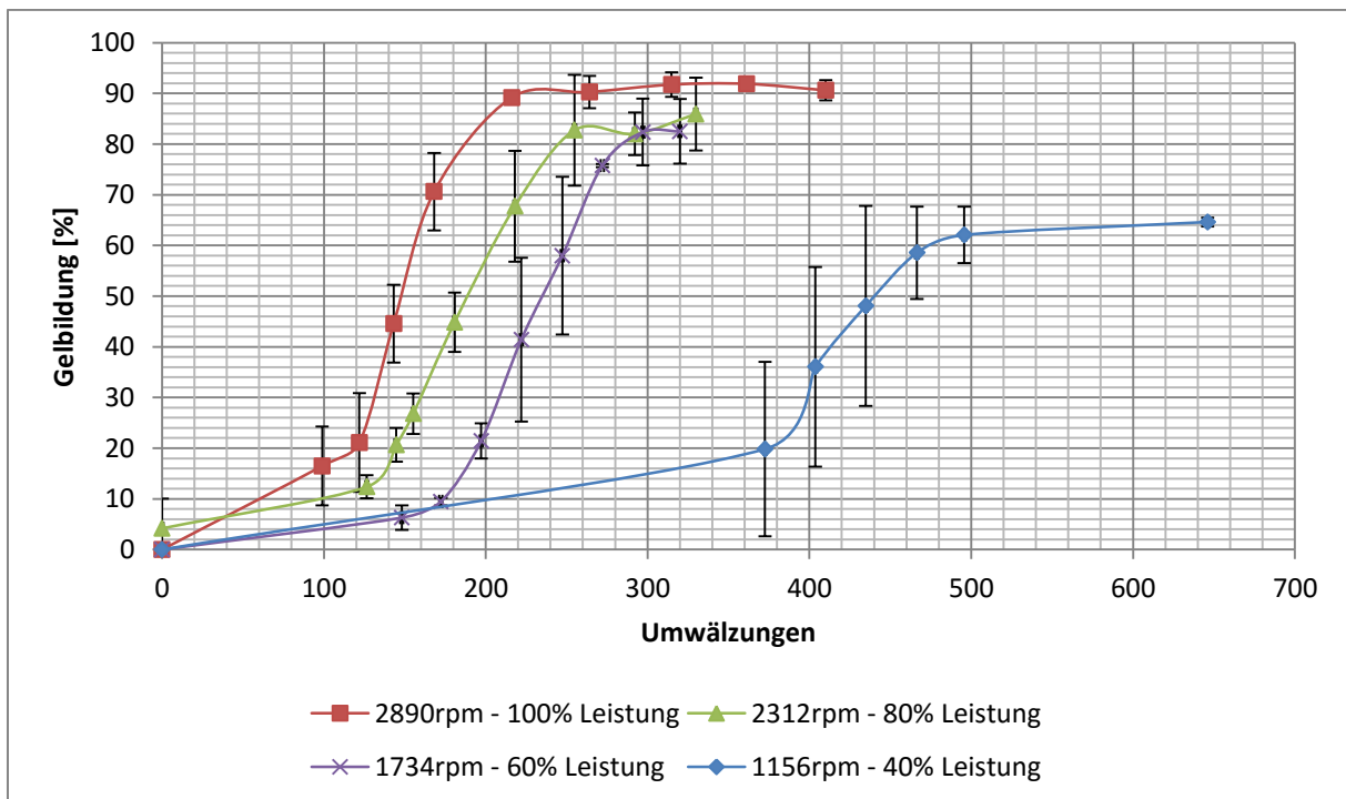
Abbildung 36: Verschiedene über den Frequenzumrichter eingestellte Betriebspunkte der Kreiselpumpe A, Mittelwerte und Standardabweichungen, \beta -Glucan-Charge #B02
