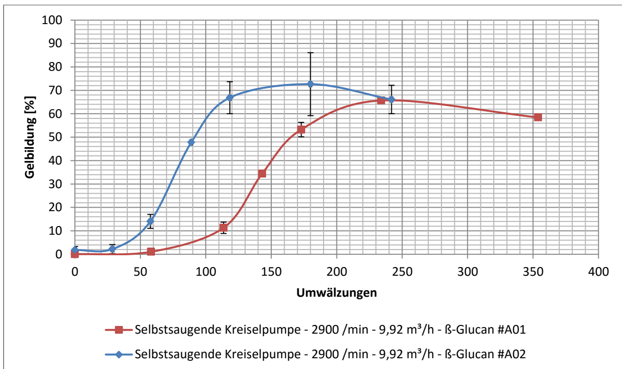
Abbildung 19: Gelbildungskurven der selbstsaugenden Kreiselpumpe bei 2900 \text{ min}^{-1} bei gleichen Versuchsbedingungen mit unterschiedlichen \beta -Glucan-Chargen, Mittelwerte und Standardabweichungen
