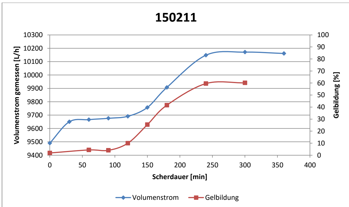
Abbildung 40: Volumenstrom und Gelbildung – normalsaugende Kreiselpumpe A, nominaler Betriebspunkt, \beta -Glucan-Charge #A02
