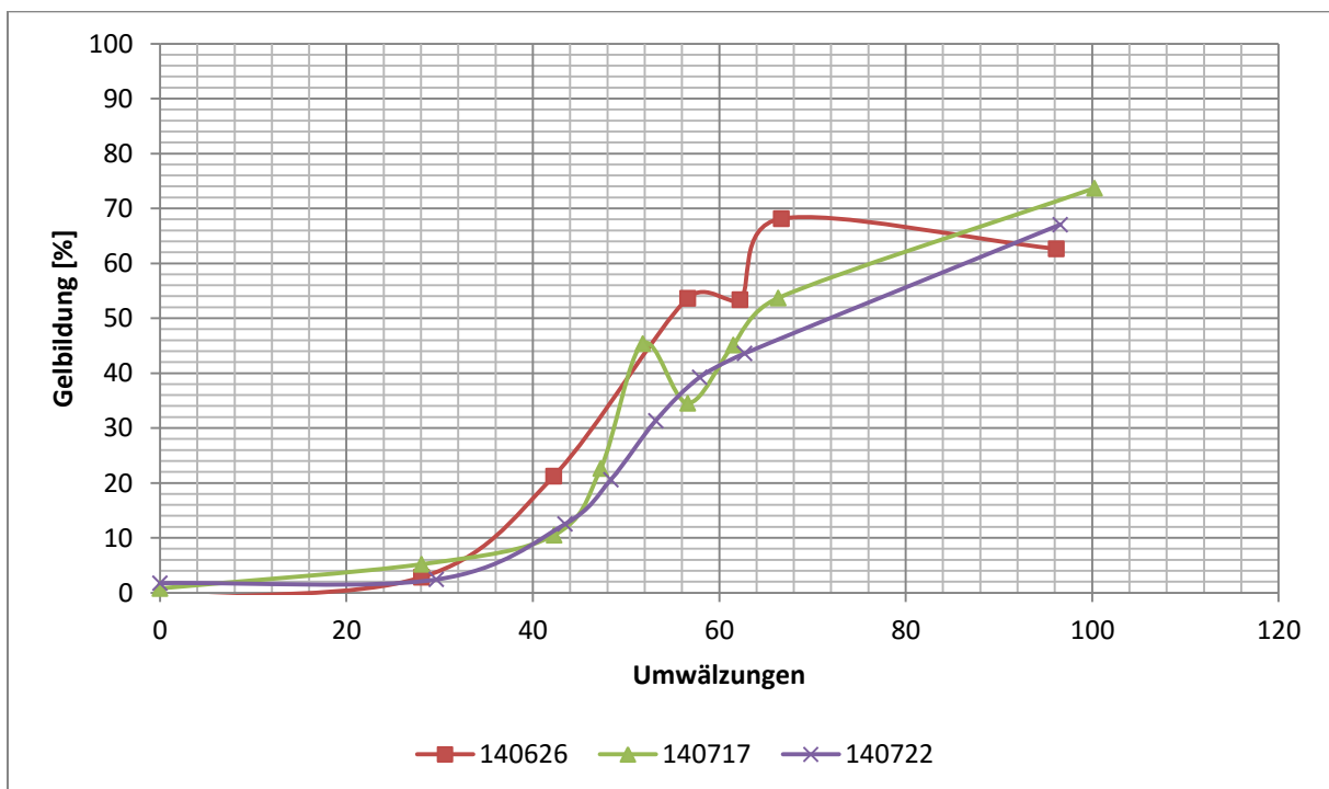
Abbildung 15: Gelbildungskurven der Scherkraftmischpumpe der drei Versuche bei 2400 min -1
