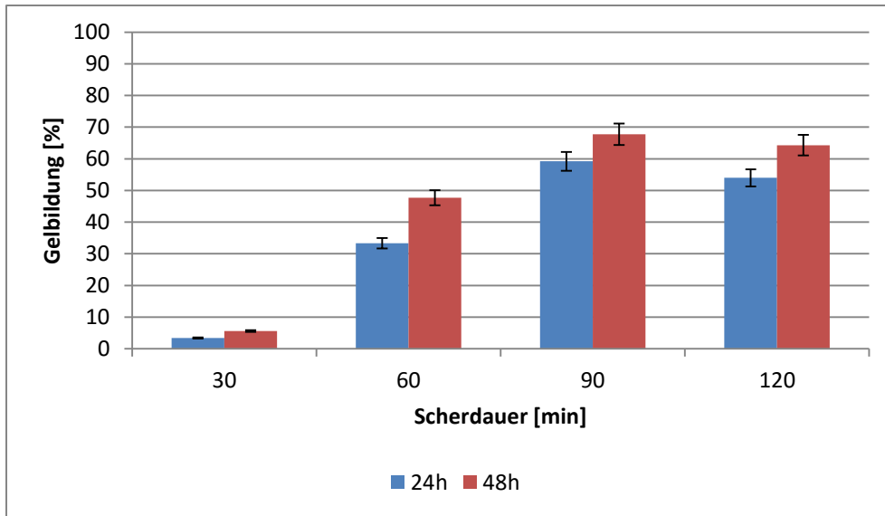
Abbildung 3: Abhängigkeit der \beta -Glucan-Gelbildung von der Lagerdauer bei gleicher Konzentration und Scherstärke, n = 3
