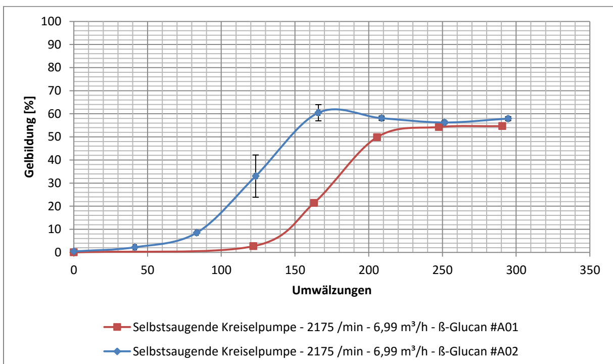
Abbildung 20: Gelbildungskurven der selbstsaugenden Kreiselpumpe bei 2175 \text{ min}^{-1} bei gleichen Versuchsbedingungen mit unterschiedlichen \beta -Glucan-Chargen, Mittelwerte und Standardabweichungen
