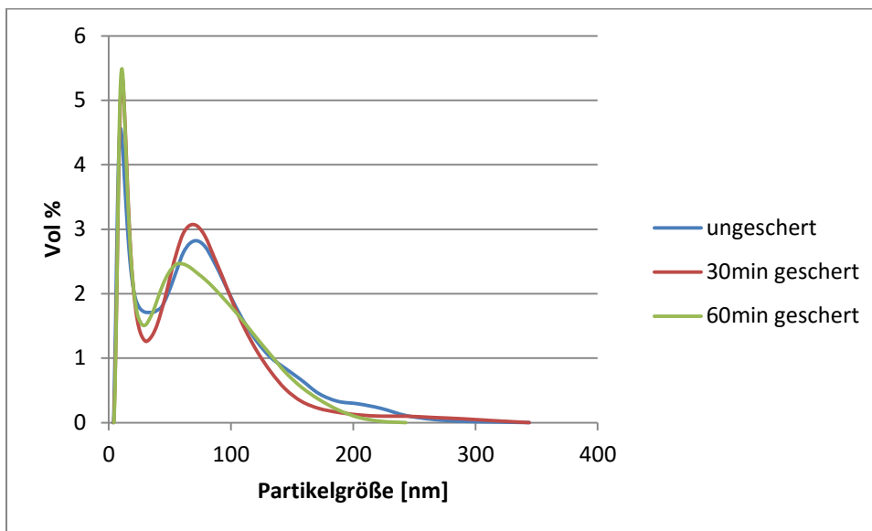
Abbildung 7: Partikelgrößenverteilung in 10 prozentiger Kieselollösung nach 0 Minuten, 30 Minuten und 60 Minuten starker Scherbeanspruchung
